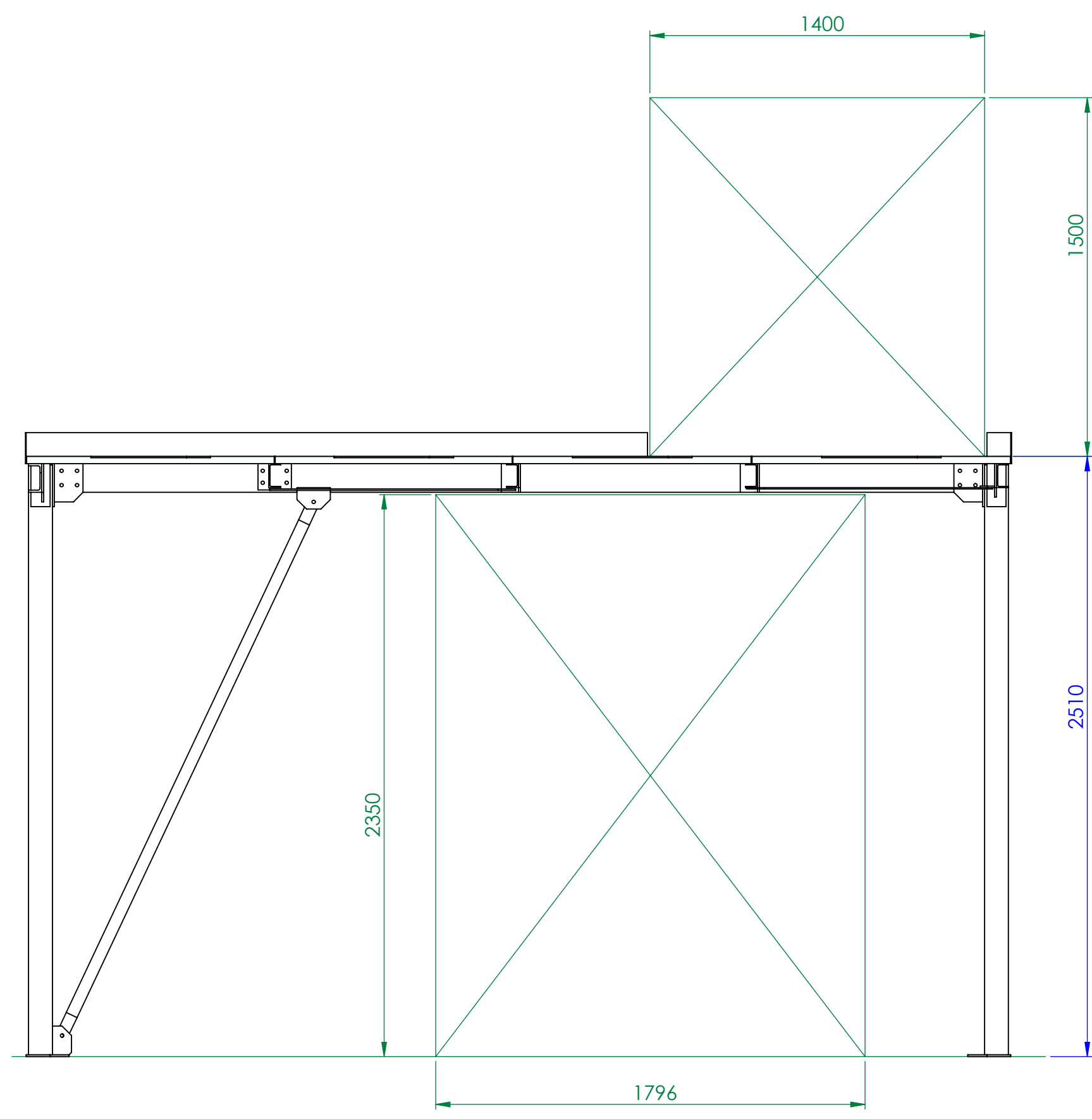
COUPE A-A
