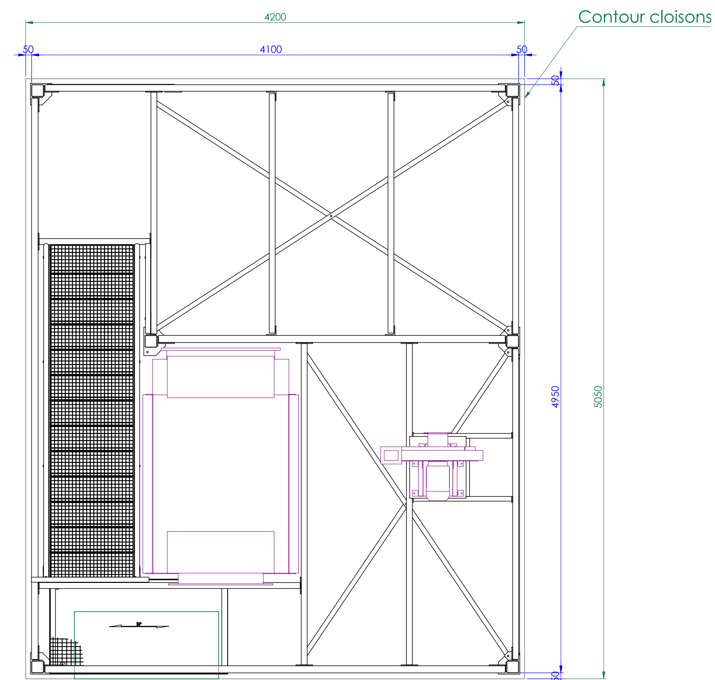
VUE DE DESSUS Sans caillebotis
